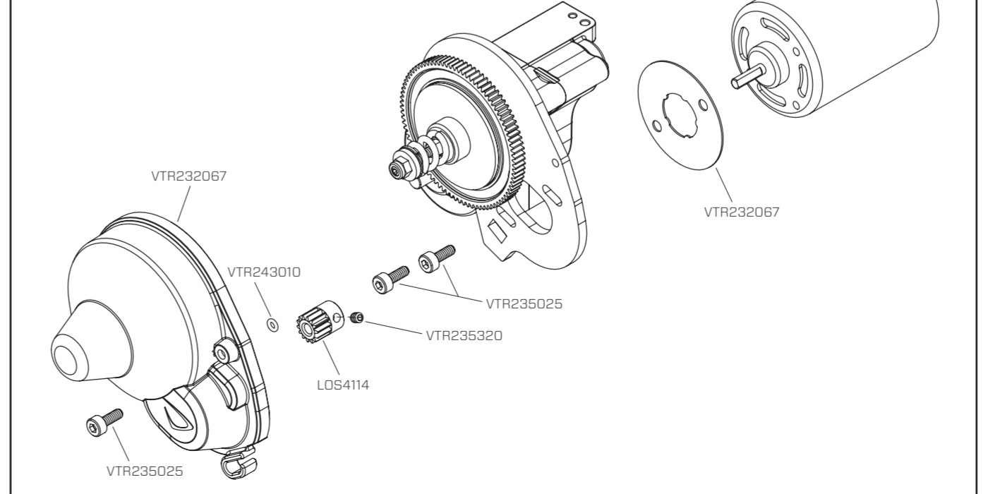
MOTOR INSTALLATION MOTOREINBAU INSTALLATION DU MOTEUR INSTALLAZIONE DEL MOTORE
