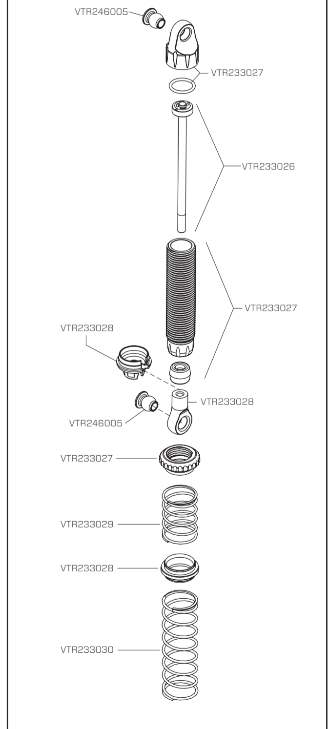
SHOCK ASSEMBLY STOßDÄMPFER MONTAGE ASSEMBLAGE D'UN AMORTISSEUR GRUPPO AMMORTIZZATORE
