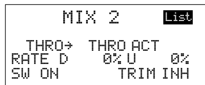
Mischfunktion 2 (Seite 125)
